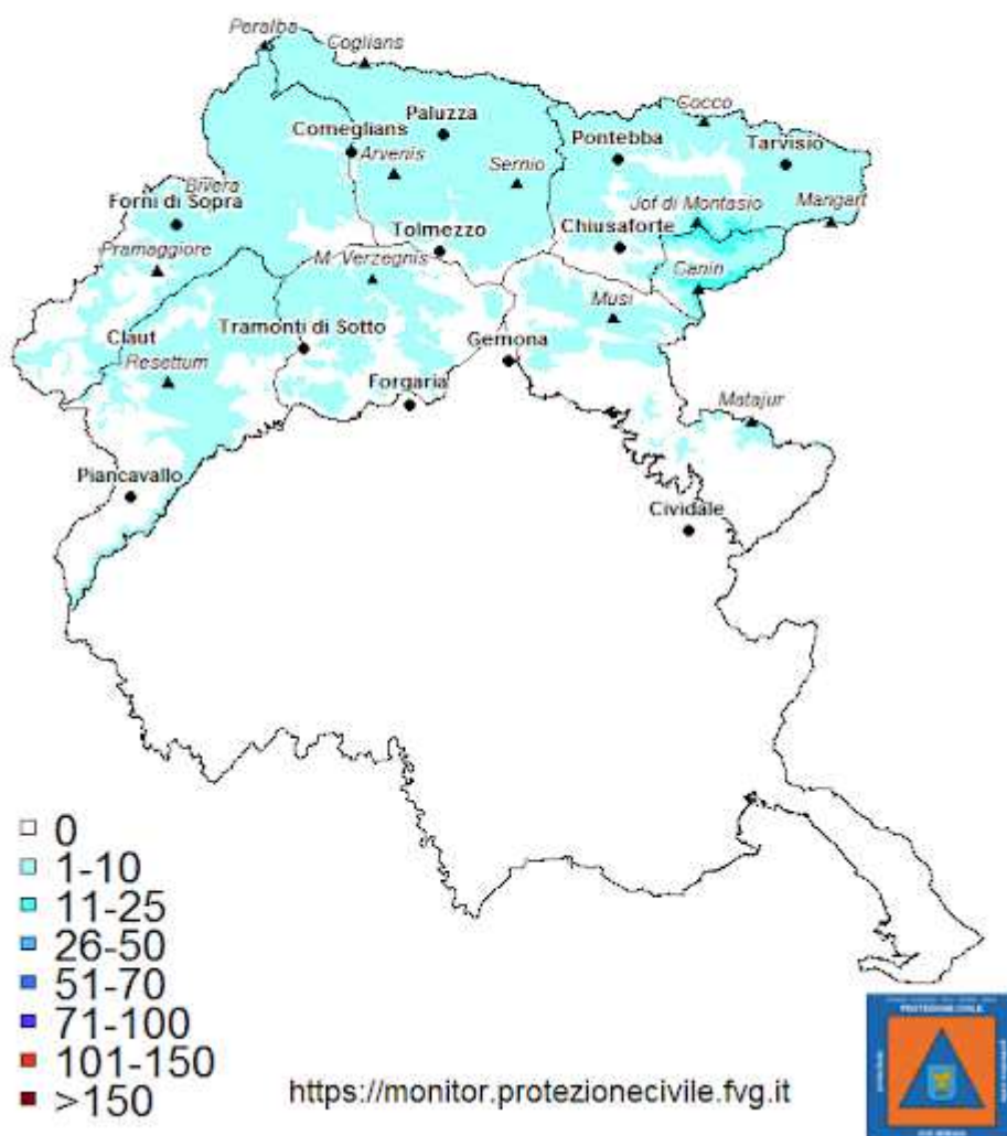
Figura 2 - Mappa della neve fresca delle ultime 24 h al suolo.
